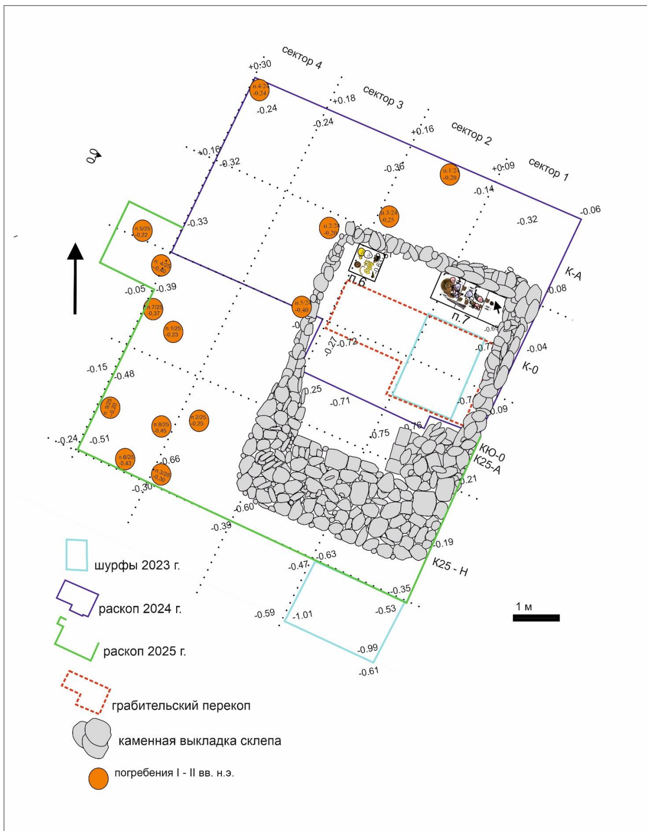
Рис. 1. План участка раскопа «Котел» по итогам работ 2023–2025 гг. Fig. 1 Excavation site plan «Kotyol» based on the results of the 2023–2025 works
